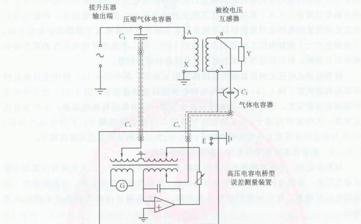
(b) 使用高压电容电桥型误差测量装置的检定线路
